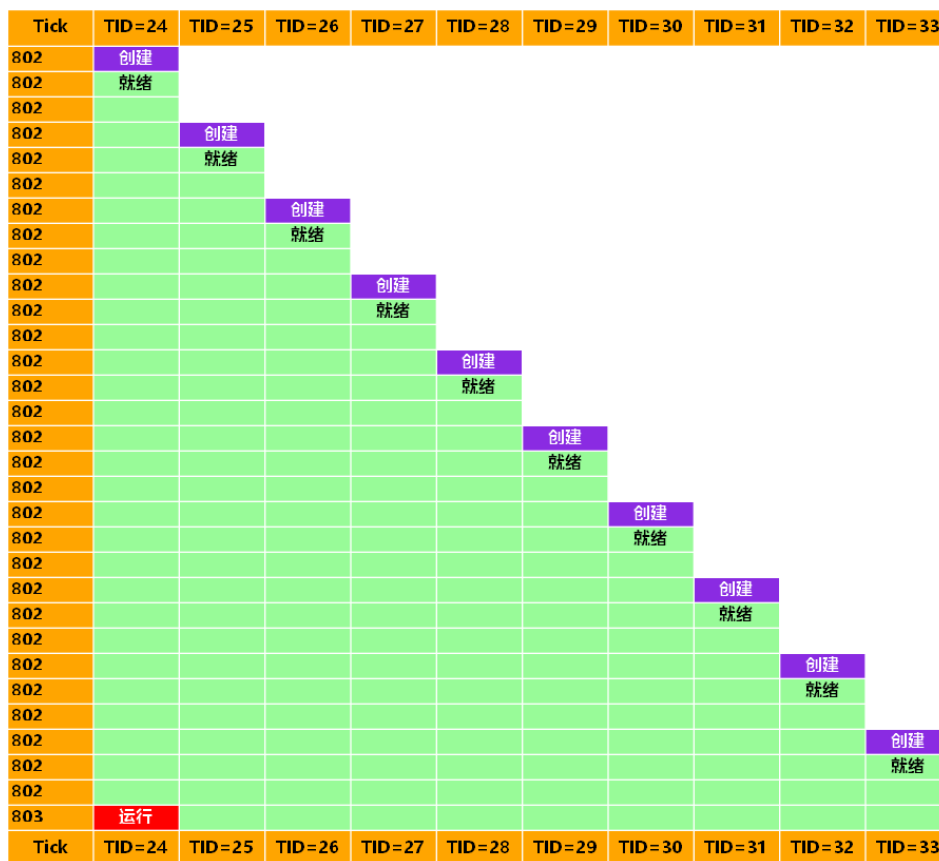
图 14-3：“rr”命令创建的 10 个线程的运行轨迹
