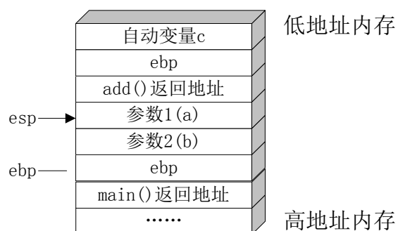
图 2-12: RET 指令执行后的堆栈状态
