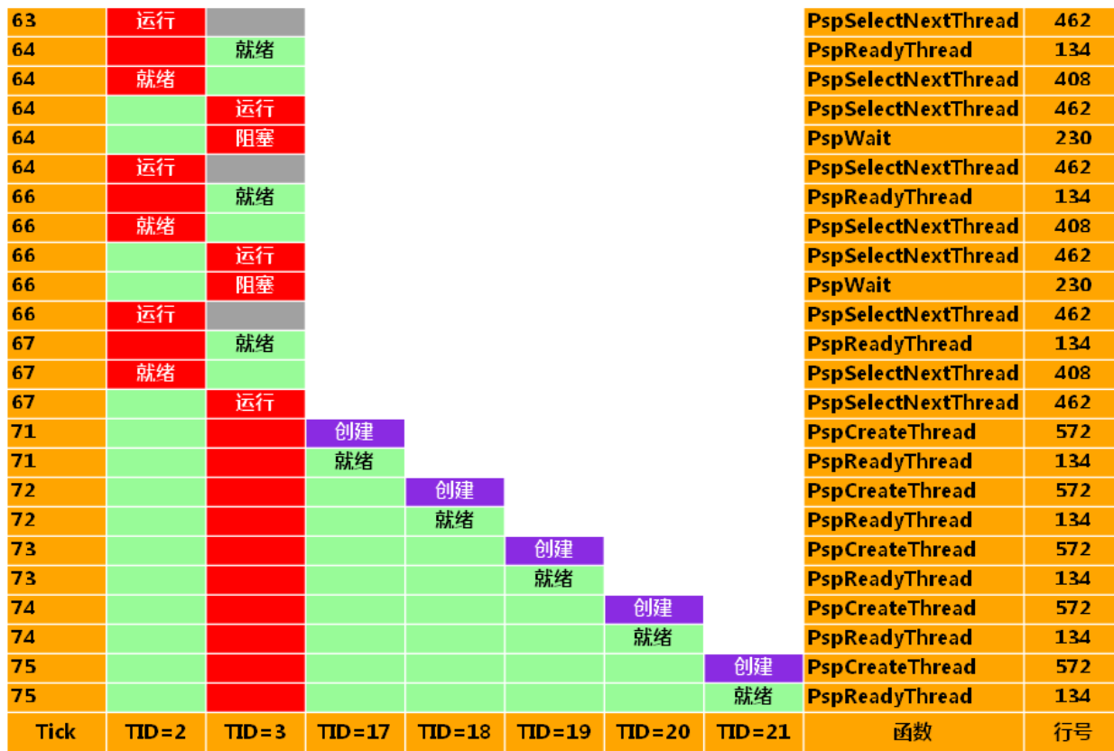
图 11-20：系统线程的运行轨迹
