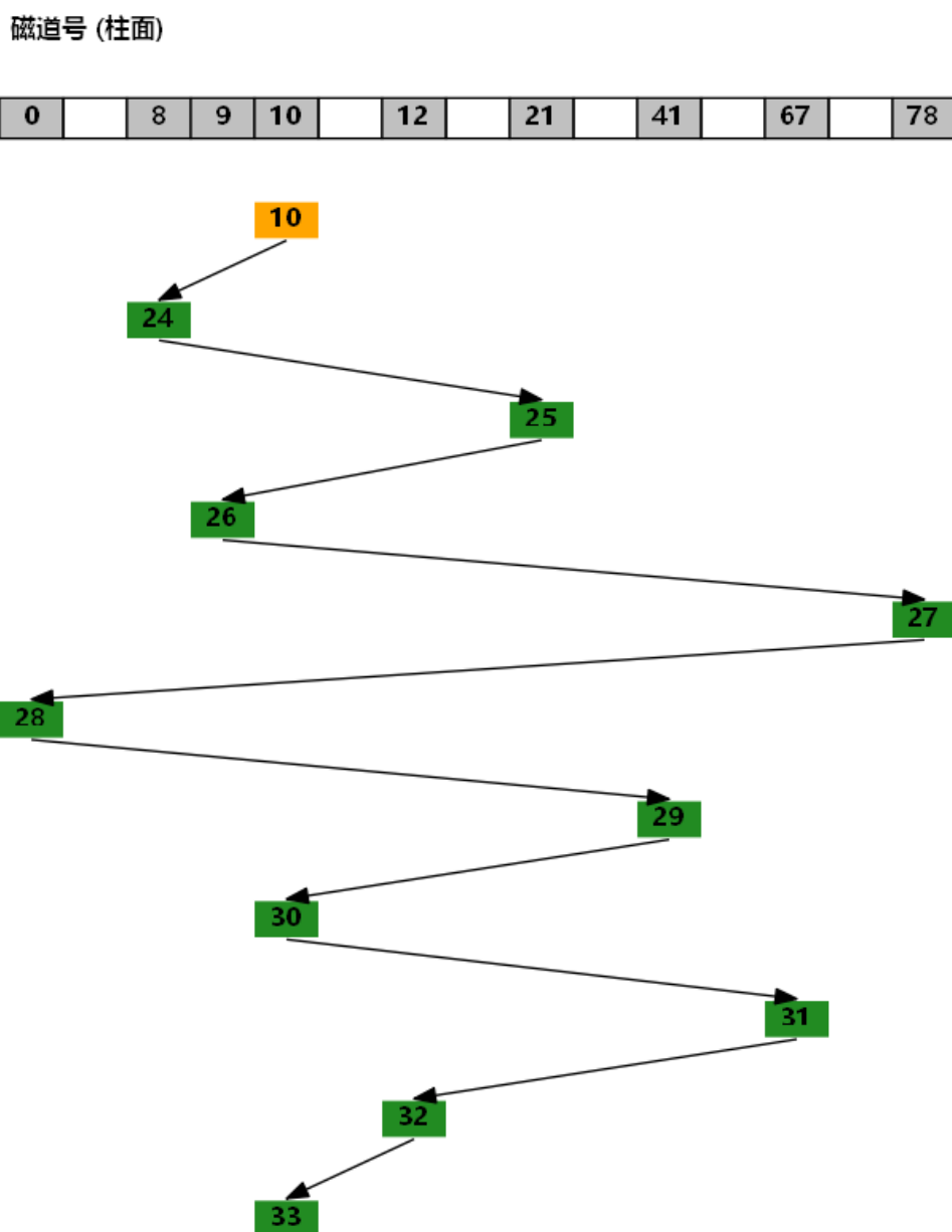
图 19-2: FCFS 算法磁头移动的轨迹
