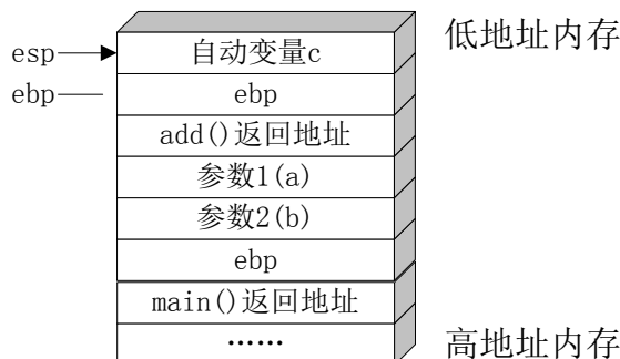
图 2-10：进入函数后的堆栈状态
