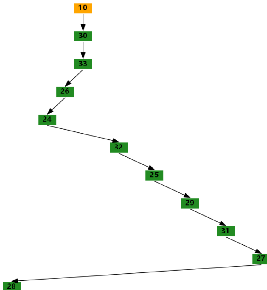
图 19-4: SSTF 算法磁头移动的轨迹
