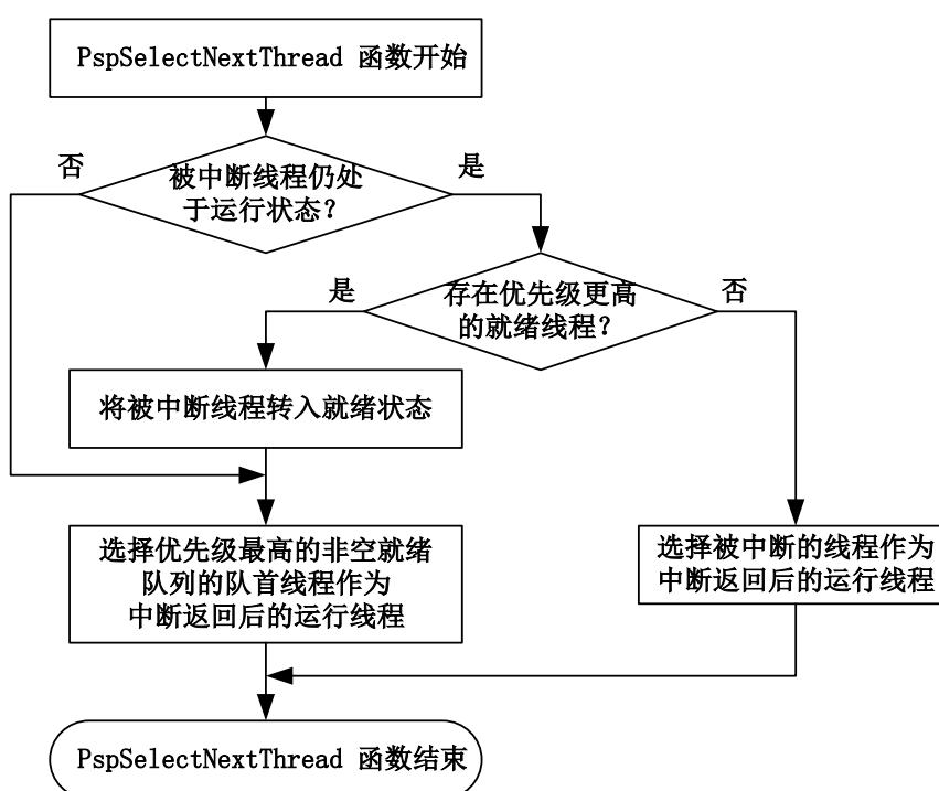
图 5-9：PspSelectNextThread 函数流程图
