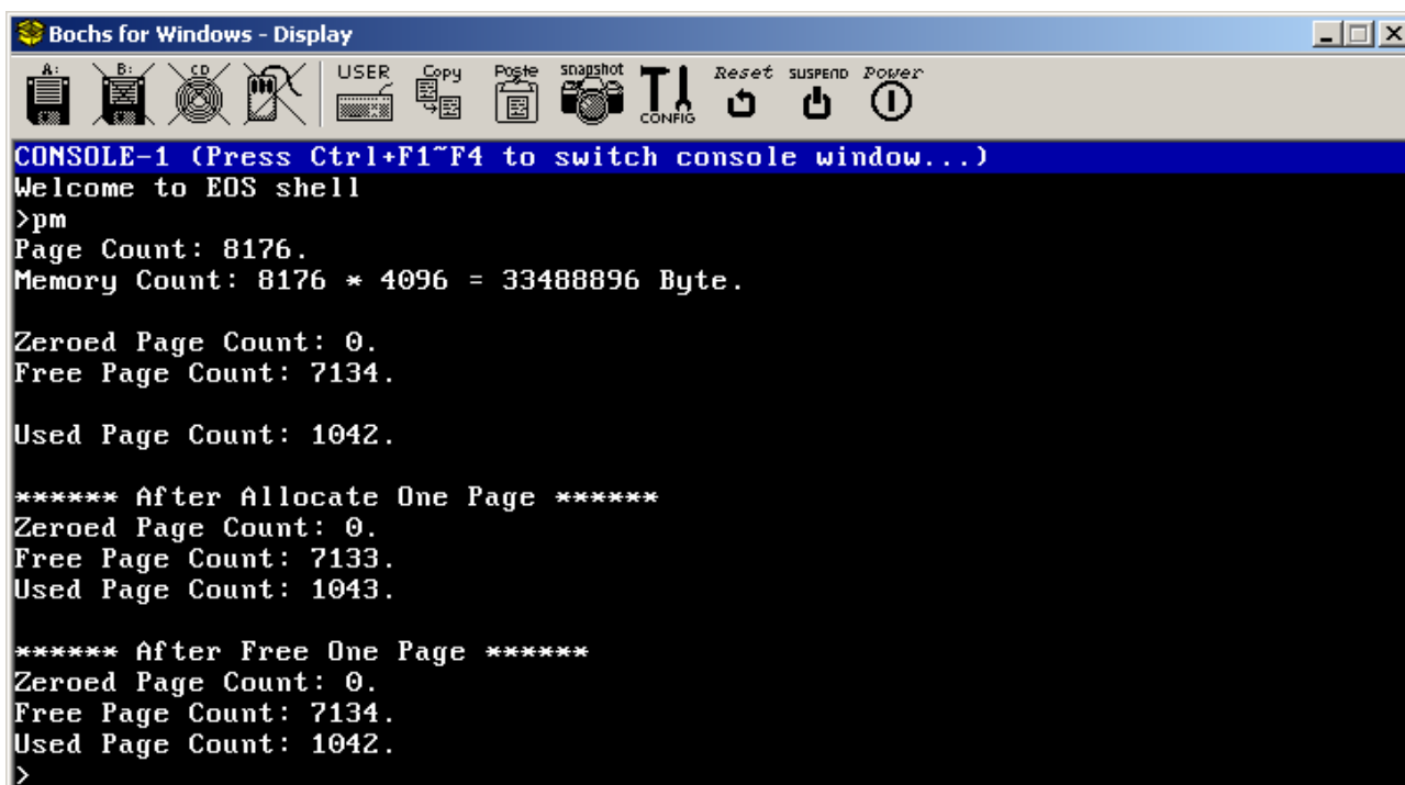
图 15-3: 分配一个物理页和释放一个物理页后物理存储器的变化情况。
