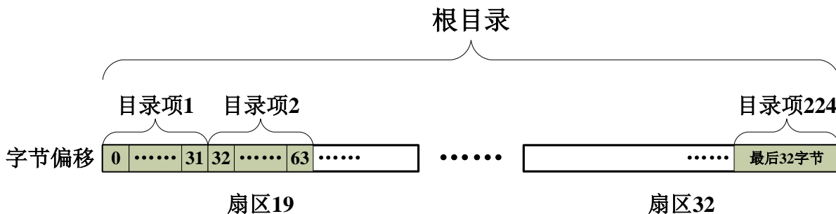
图 8-4：目录项在根目录中的分布
