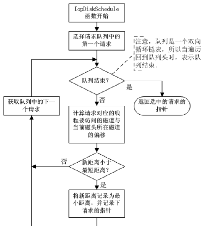
图 19-3: 实现了 SSTF 算法的 IopDiskSchedule 函数流程图
