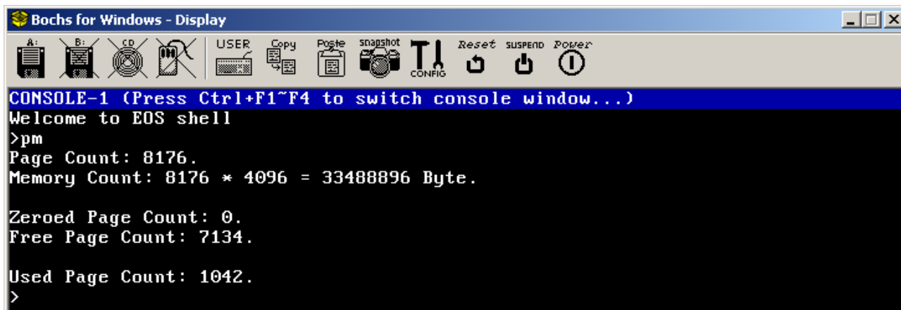
图 15-2: “pm” 命令的执行结果
