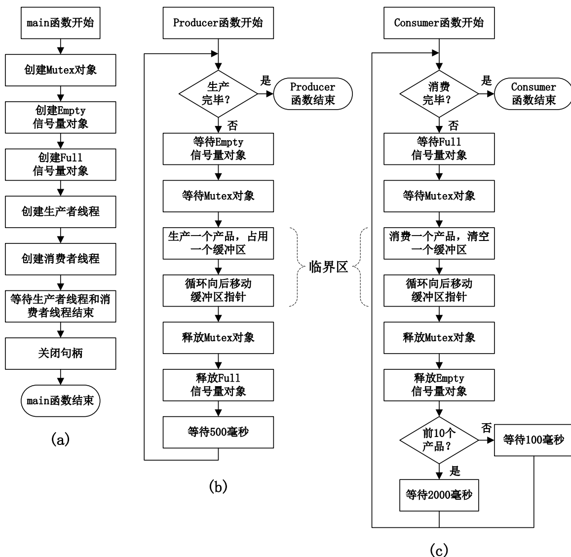
图 13-1: (a)main 函数流程图; (b)Producer 函数流程图; (c)Consumer 函数流程图
