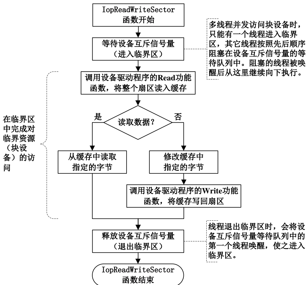
图 7-2: IopReadWriteSector 函数流程图
