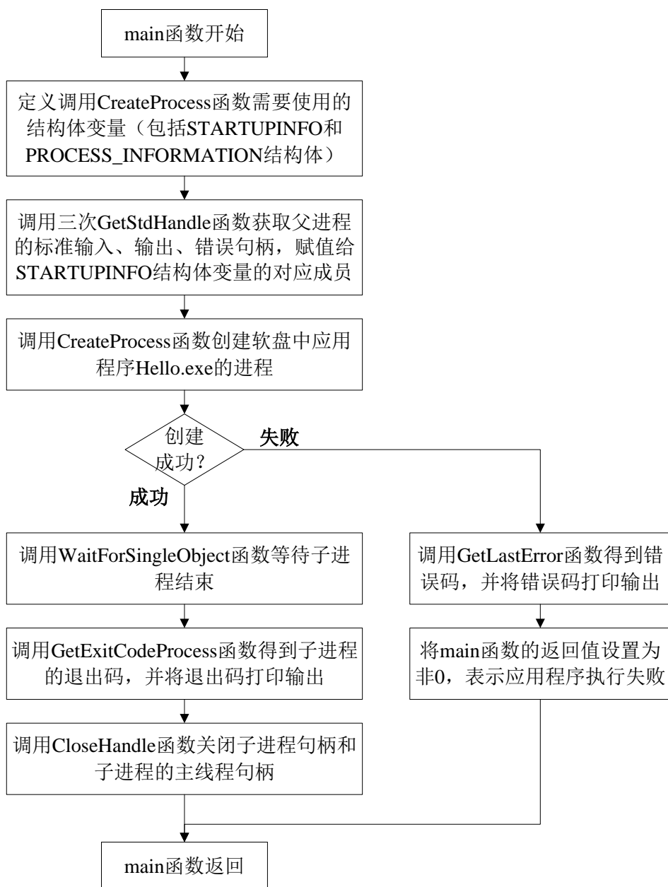
图 11-3: main 函数流程图
