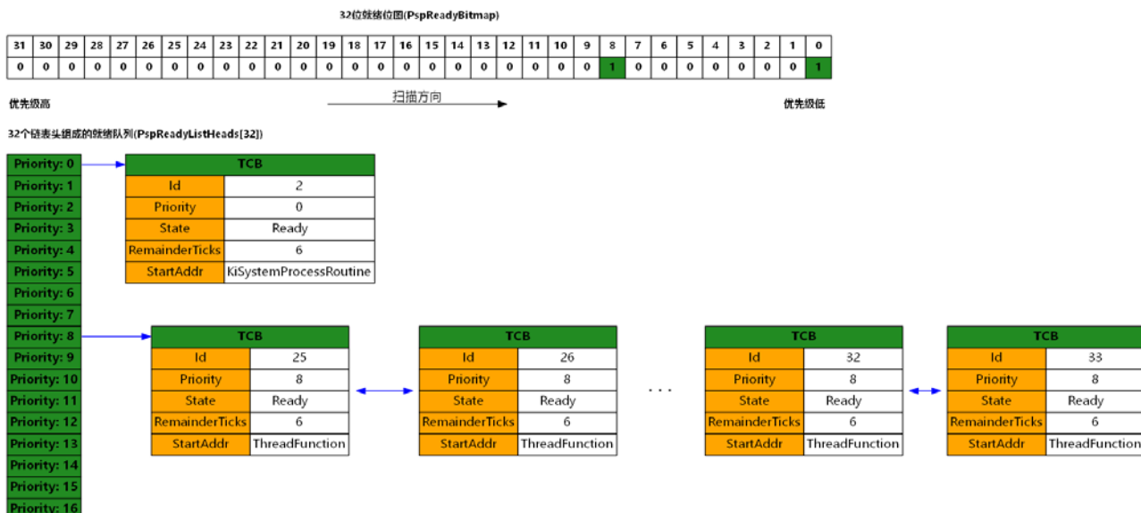
图 14-4：“rr”命令创建的 10 个线程有 9 个在就绪线程队列中
