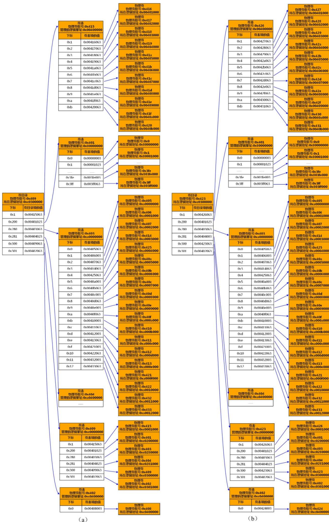
图 16-3: (a) 应用程序进程一的二级页表映射 (b) 应用程序进程二的二级页表映射
