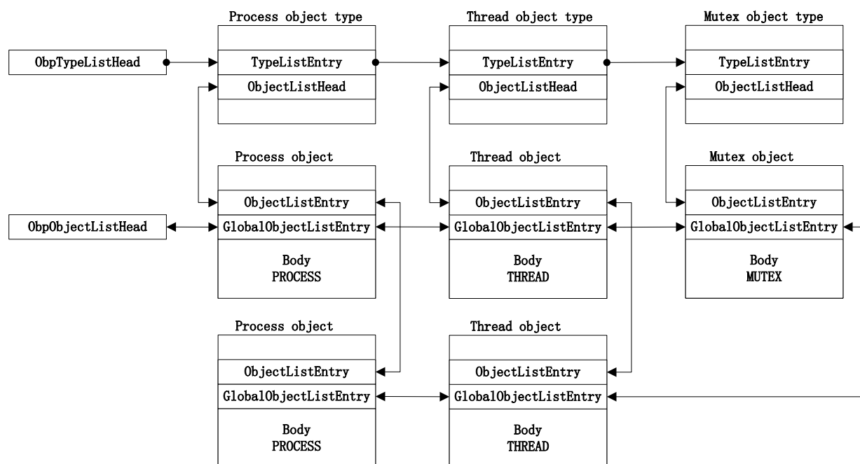
图 4-2：对象类型和对象组成的链表。
