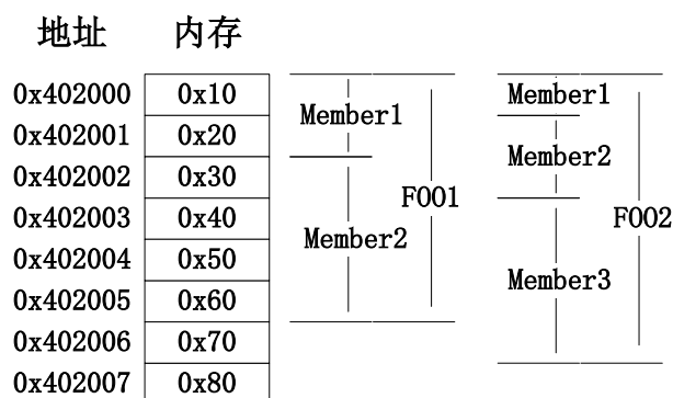
图 2-16：按照 1 字节对齐后的结构体的内存布局。
