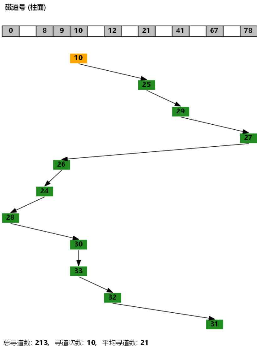
图 19-8: N 值取 6 时, N-Step-SCAN 算法磁头移动的轨迹
