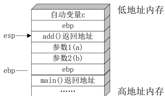
图 2-11: LEAVE 指令执行后的堆栈状态
