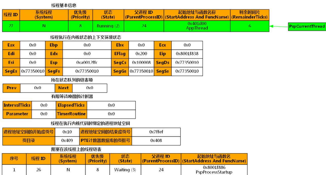
图 11-14: 工作线程的线程控制块
