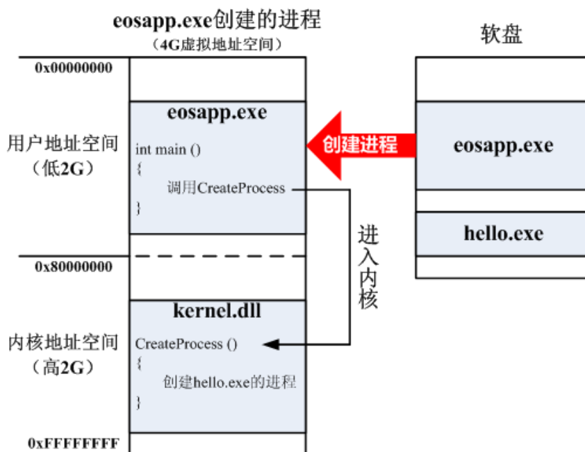
图 11-7: EOS 应用程序 eosapp.exe 创建的进程
