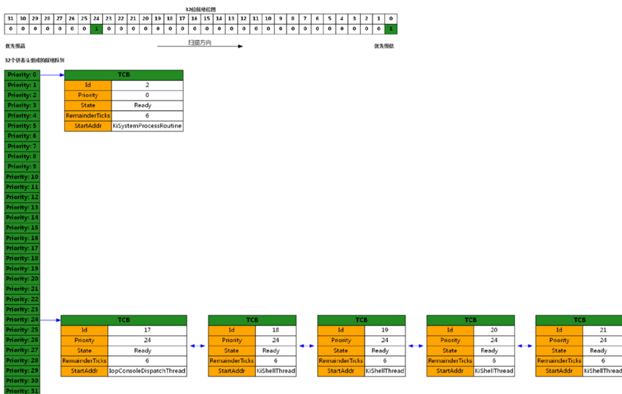
图 11-19：就绪线程队列
