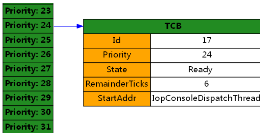
图 12-3：控制台派遣线程进入就绪状态后挂接在优先级为 24 的就绪队列中
