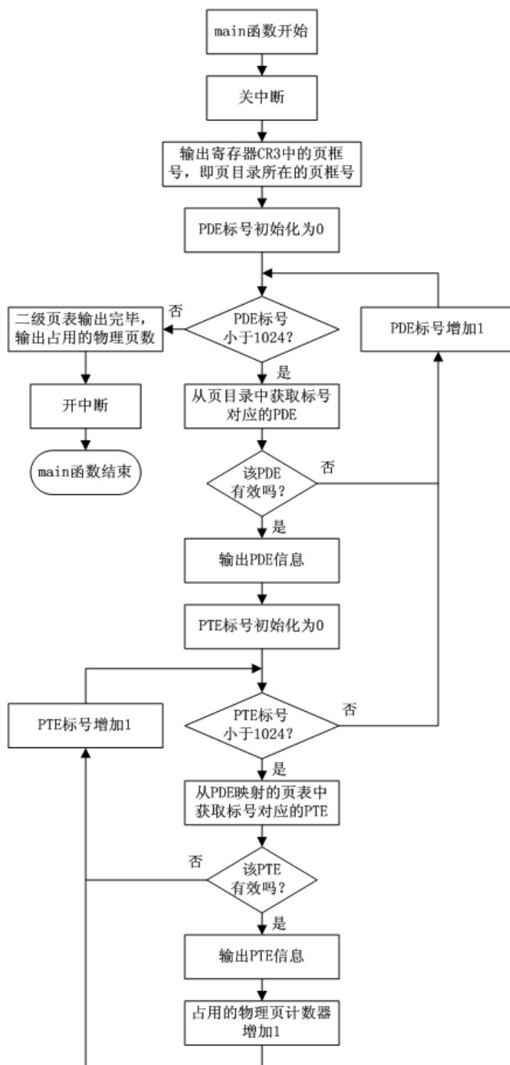
图 16-1: main 函数流程图
