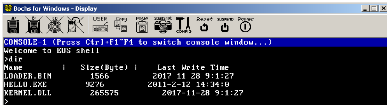
图 21-2：“dir”命令的执行结果
