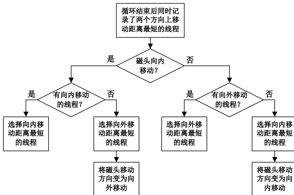
图 19-6：循环结束后，根据磁头移动方向选择合适线程的流程图
