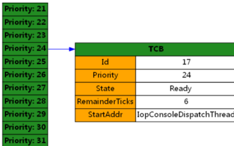
图 14-6：控制台派遣线程进入就绪队列
