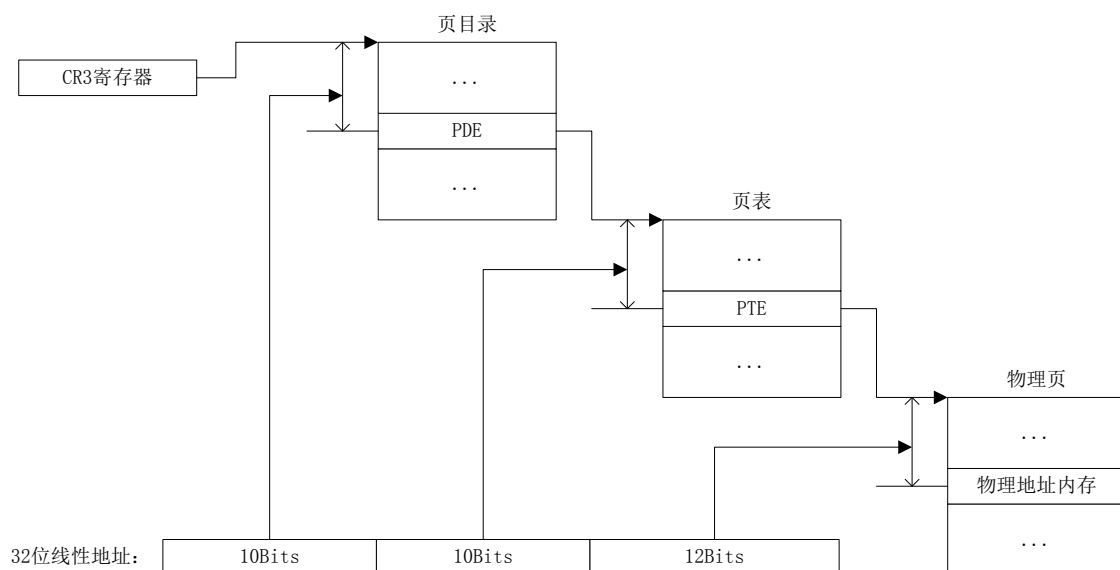
图 6-1：二级页表分页机制
