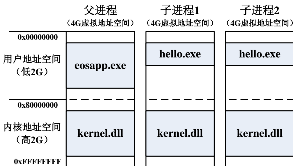
图 11-12：同时创建一个应用程序的多个进程
