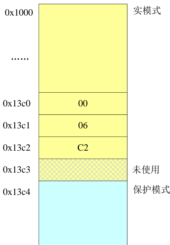
图 10-4: Loader 程序在内存中的布局
