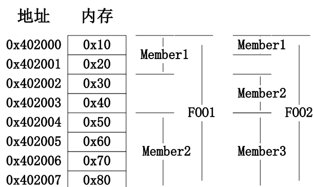
图 2-15：默认情况下结构体的内存布局。
