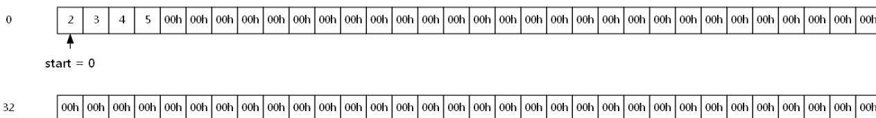
图 18-4: 需要从串口发送的数据被放入串口设备的发送缓冲区
