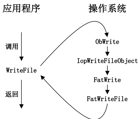
图 8-16：写文件相关函数的调用流程。
