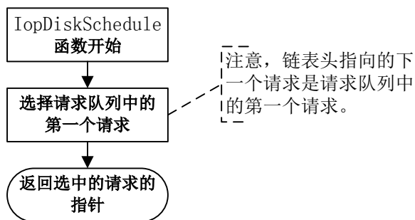
图 19-1: 实现了 FCFS 算法的 IopDiskSchedule 函数流程图
