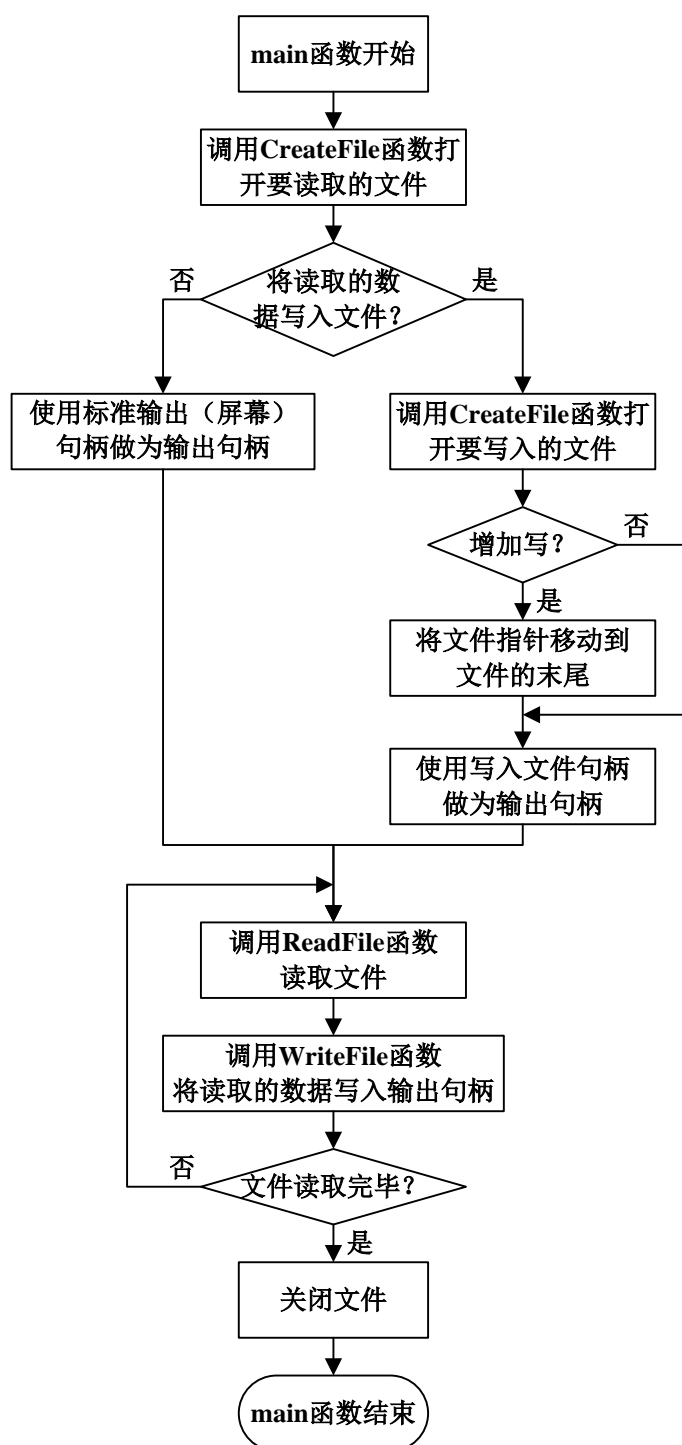
图 22-1: main 函数流程图
