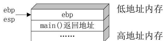
图 2-8：初始的堆栈状态
